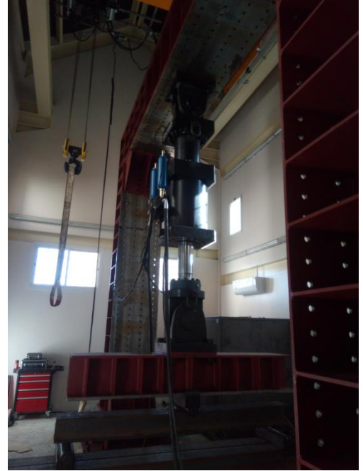
شكل 1 ماكينة اختبار المنشآت
